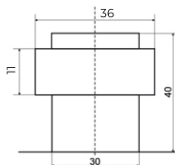
Vettore 014 AB (бронза)
